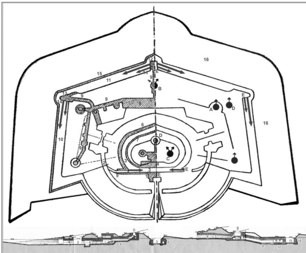
1 - corp de gardă redus, 2 - corp de gardă fort, 3 - șanț redus, 4 - local redus, 5 - cazemată de contraescarpă, 6 - galerie de contraescarpă, 7 - escarpă zidită, 8 - local fort, 9 - potemă, 10 - șanț lateral, 11 - șanț anterior, 12 - caponieră dublă, 13 - semicaponieră, 14 - șanț diamant, 15 - contraescarpă zidită, 16 - glacis A - cupolă Montluçon cu un obuzier de 210 mm, model 1891 (2x), B - cupolă St. Chamond cu două tunuri de 150 mm, model 1891 (1x), C - cupolă Montluçon cu două tunuri de 150 mm, model 1891 (2x), D - turelă cu eclipsă cu un tun de 57 mm (5x), E - tun de 57 mm, pentru flancarea șanțurilor (13x)
